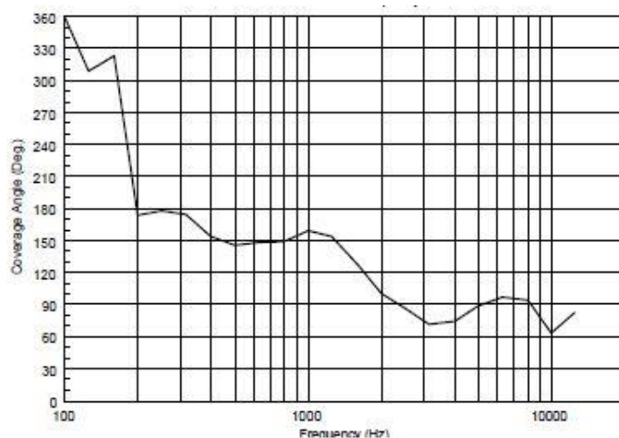
Vyžarovací uhol v závislosti od frekvencie
