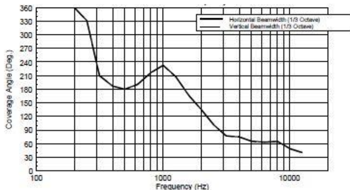
Vyžarovací uhol v závislosti od frekvencie
