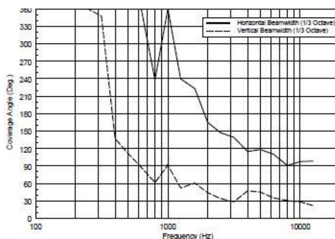
Vyžarovací uhol v závislosti od frekvencie
