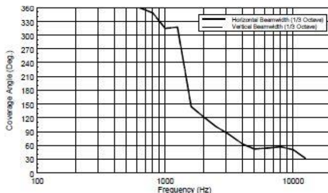
Vyžarovací uhol v závislosti od frekvencie
